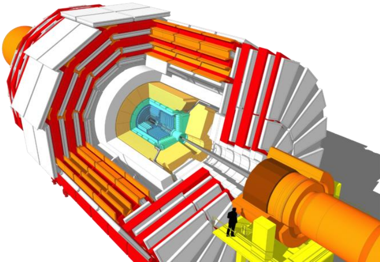
لایه‌های متحدالمرکز آشکارساز اطلس؛ طول: ۴۵ متر، ارتفاع: ۲۵ متر
